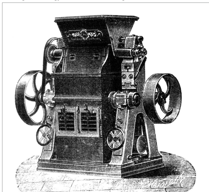
Kéthengeres Ganz gyári Mechwart-féle hengersizék
