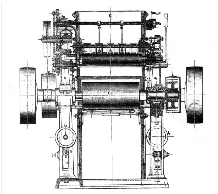
Két pár hengerrel készült hengersizék metszete
