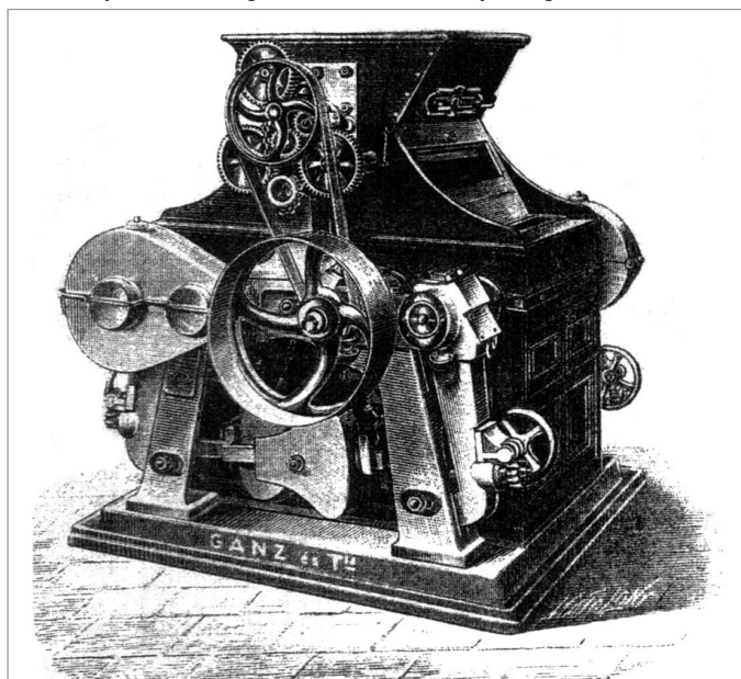
Faszekrényes kettős hengersizék 200 mm átmérőjű hengerrel
